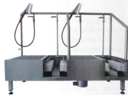
Aschl: Doppel-Stiefelwaschanlage.
